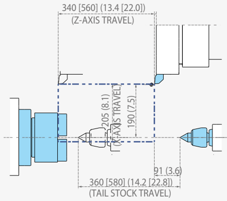
OD Holder
